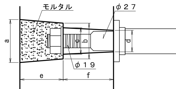
AS 柵ステップ穴形状寸法表
