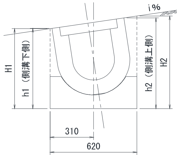
勾配対応寸法早見表 ( 300×300の場合 )
