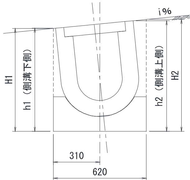
勾配対応寸法早見表 (300×400の場合)
