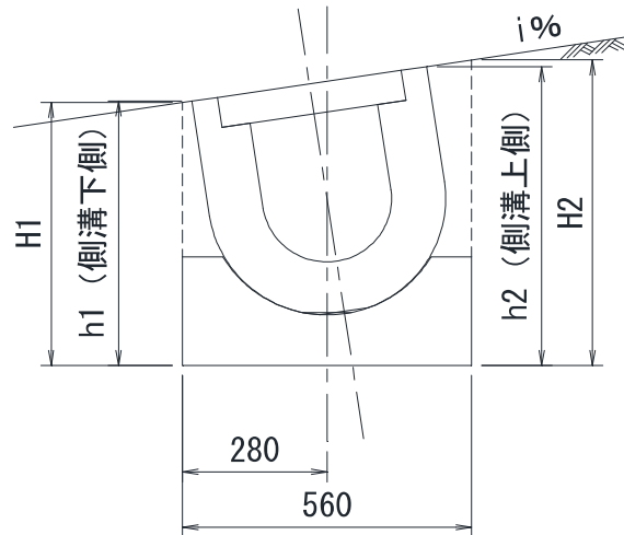
勾配対応寸法早見表 (250×250の場合)
