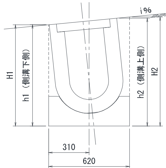
勾配対応寸法早見表 (300×500の場合)
