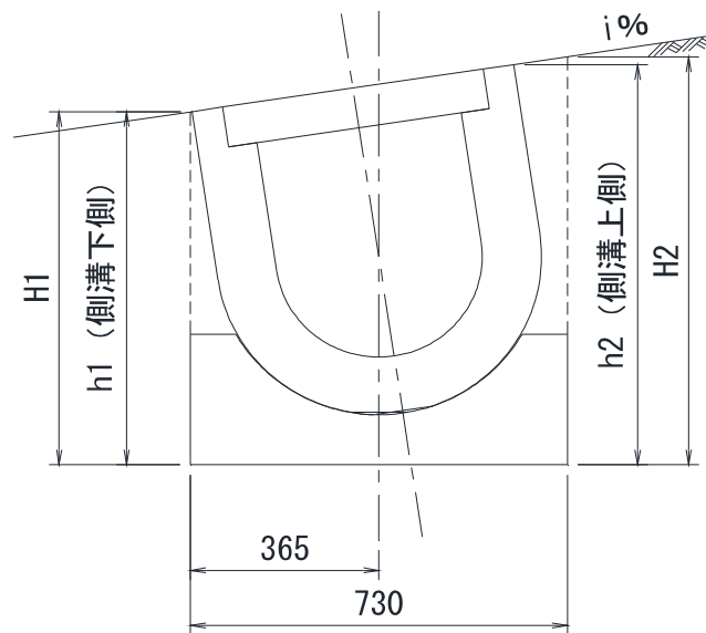
勾配対応寸法早見表( 400×400の場合)
