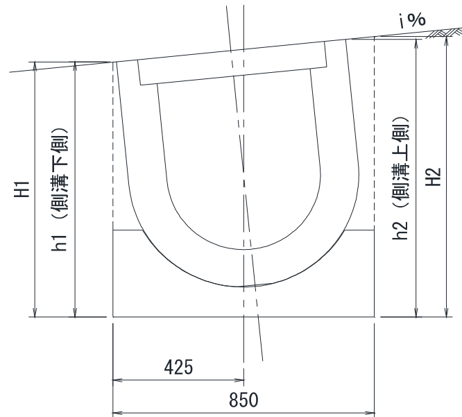
勾配対応寸法早見表( 500×500の場合)
