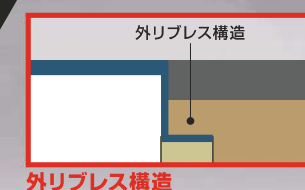
外リブレス構造
